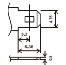
F1 (FASTON TAB 187)
